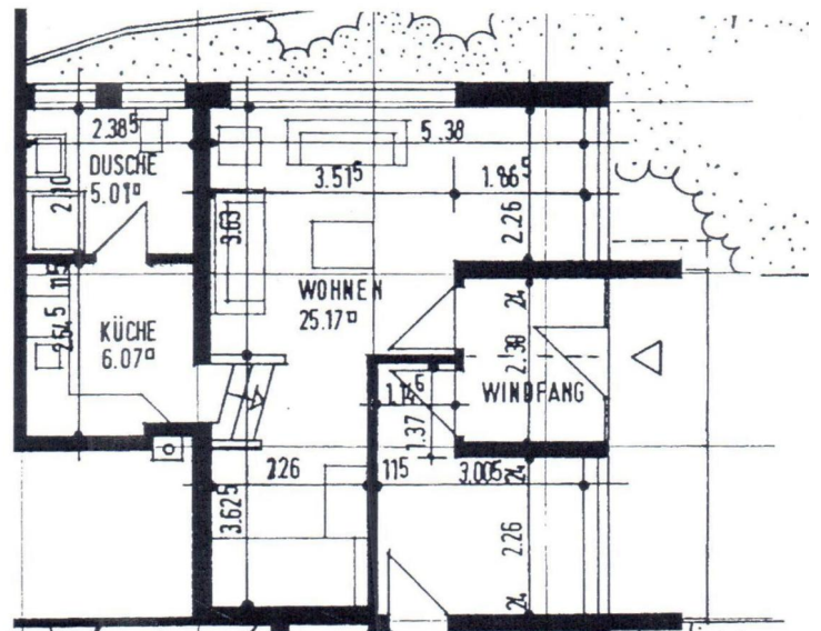
Grundrissplan:
